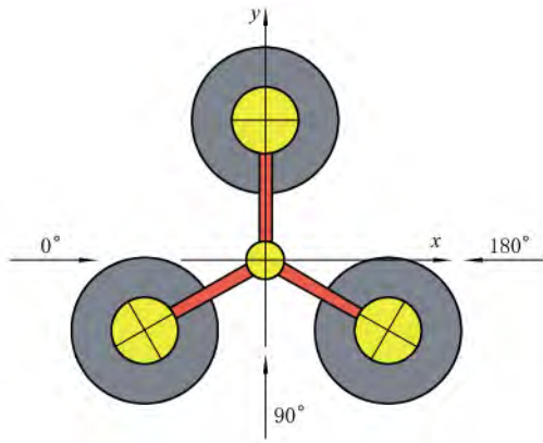
图 2 浮式平台的平面坐标系
