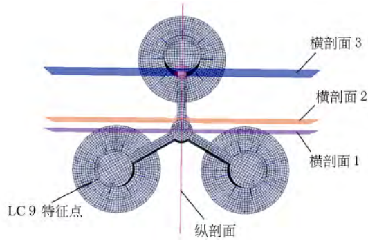
图 4 强度分析的剖面 and 节点
