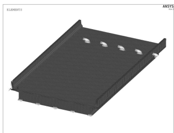
图 4 桥梁有限元模型 Fig.4 The bridge finite element model
