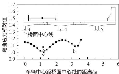
图 6 弯曲应力相对值随车辆横向加载位置的变化曲线 (五梁式 T 梁桥-主梁之间刚接)
