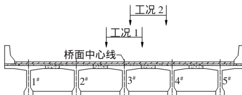
图 7 两种典型加载工况
