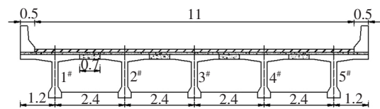
图1 桥梁典型横断面(单位:m)
